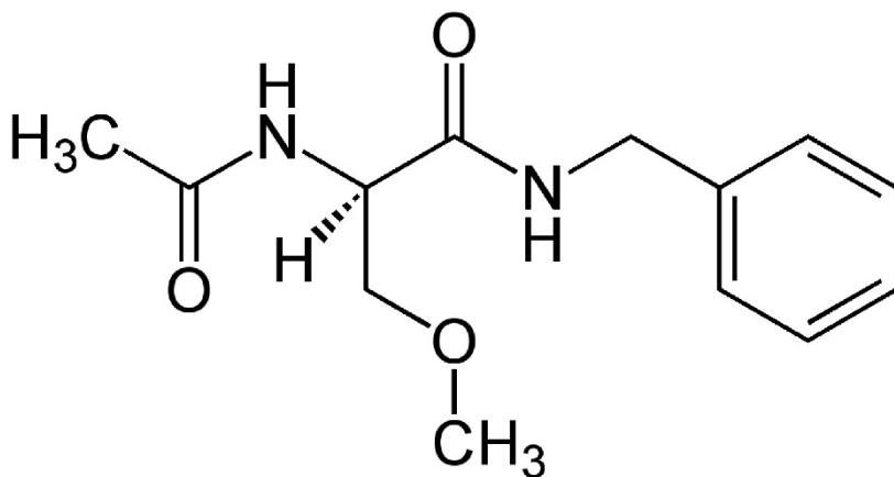
Figura 8. Lacosamida. R -enantiómero de 2-acetoamido- N -benzyl3- methoxypropionamida ( \text{C}_{13}\text{H}_{18}\text{N}_2\text{O}_3 )
