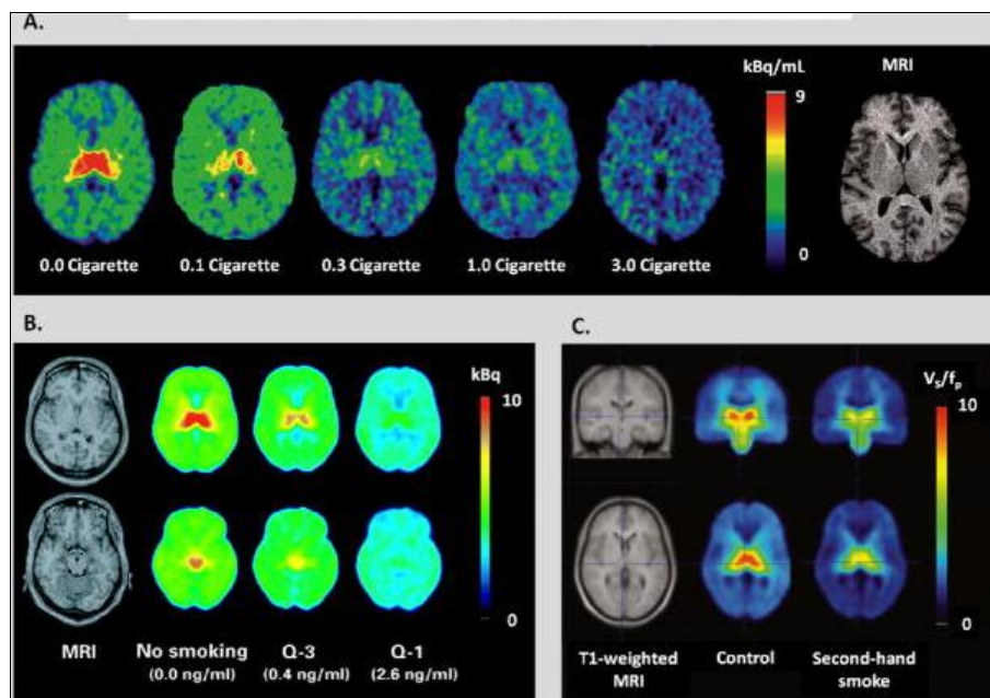
Figura 21. Ocupancia de receptores colinérgicos tras la exposición a humo de cigarrillo usando 2-FA-PET. Estudio de PET con 2- ^{18}\text{F} fluor-3-(2(S)-azetidil-metoxi) piridina (abreviado como 2-FA) de la imagen de la ocupancia de receptores nicotínicos de acetilcolina \alpha_4\beta_2^* por exposición al humo del tabaco en humanos in vivo. (A) Cortes horizontales a través del tálamo muestran que la ingesta de nicotina obtenida de cigarrillos fumados en cantidades usadas por fumadores cotidianos típicos ocupan casi por completo los receptores \alpha_4\beta_2^* indicando que los fumadores mantienen saturados estos receptores a lo largo de día (Modificado de ref 203). (B) Resultado de la exposición a cantidades relativamente pequeñas de nicotina en un cigarrillo sin nicotina (Q-3, 0.05 mg de nicotina) y uno bajo en nicotina (Q-1, 0.6 mg nicotina) que resulta en 26% y 79% de ocupancia de los receptores repectivamente a lo largo del tálamo (panel superior) y tronco cerebral (panel inferior) (Modificado de ref 204). (C) Resultado de la exposición a nicotina en un fumador moderado de segunda mano resultando en 19% de ocupancia de \alpha_4\beta_2^* tanto en fumadores como no fumadores expuestos (Modificado de ref 205).
